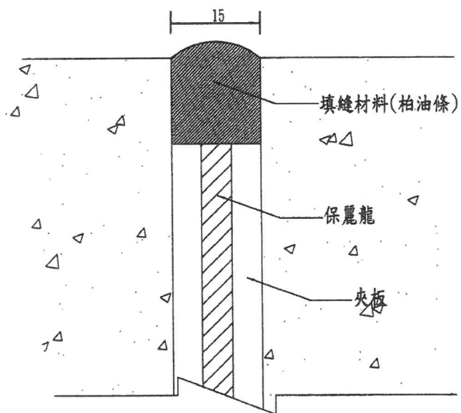
伸縮縫標準圖 比例:1/100 單位:mm
