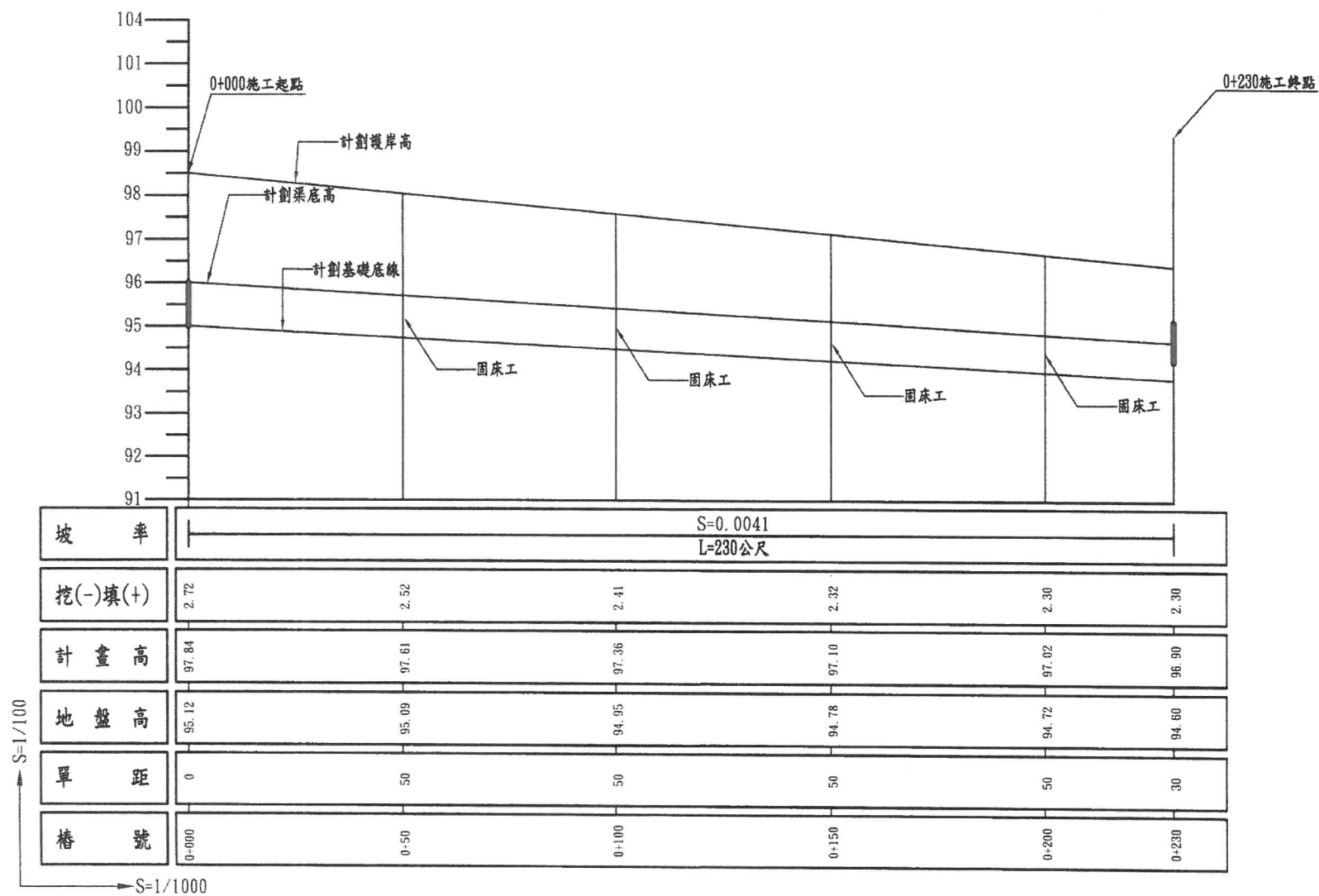
縱斷面標準圖
