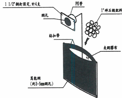
碎石濾水袋構造圖
