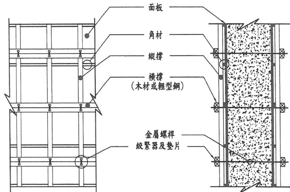
模板組立標準圖
